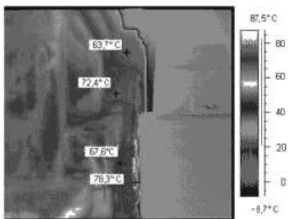
Рисунок С.4 – Редуктор со стороны входного вала
