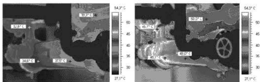
Рисунок С.10 – Термограммы двух маслоохладителей
