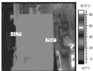
Рисунок С.3 – Двигатель и входной вал редуктора
