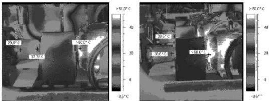
Рисунок С.9 – Термограммы насосов
